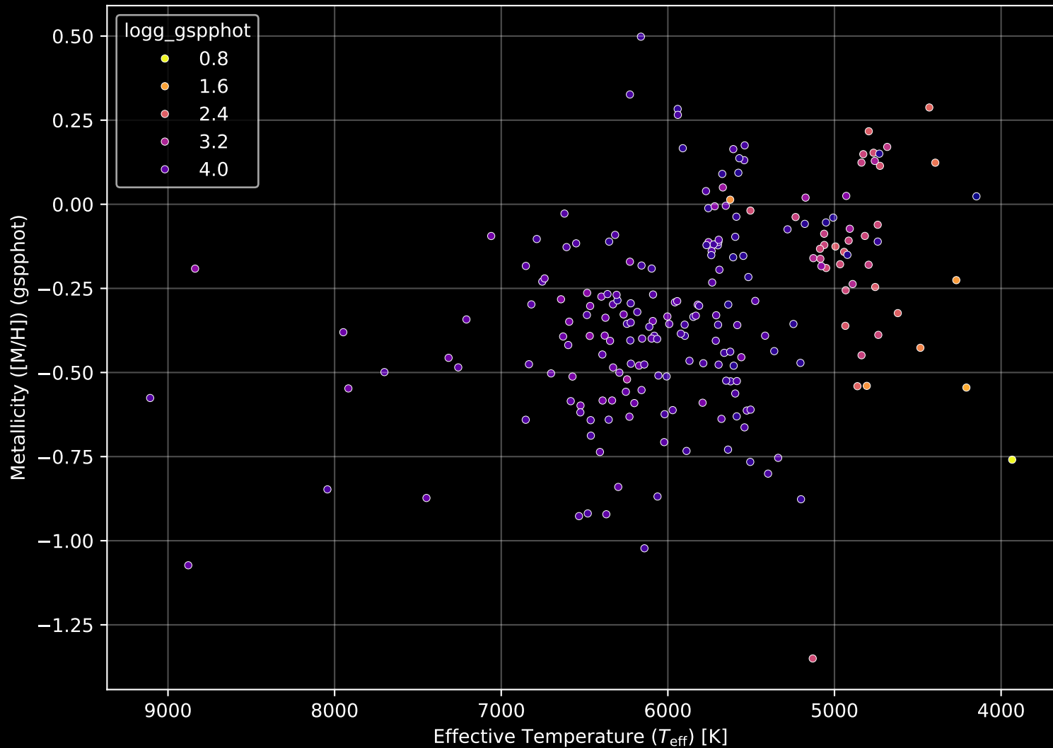
GALAH DR4 Field: [7145] Stellar Population Parameters (n= 215)
