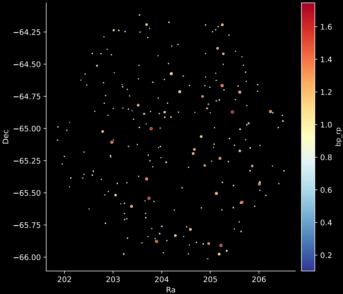
GALAH DR4 Field: [7145] Stars: 215
